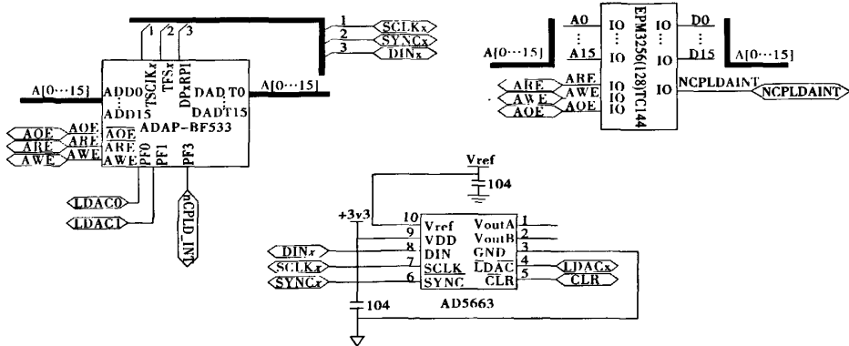
图 6 主要硬件电路
