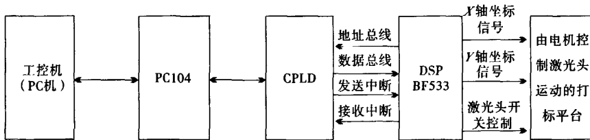
图 5 系统硬件框图
