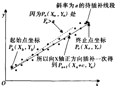
图3 插补算法示意图
