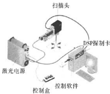
图1 系统组成图
